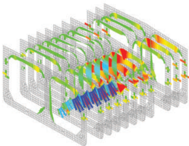
Ilustracija 4 Analiza brodske konstrukcije metodom konačnih elemenata
